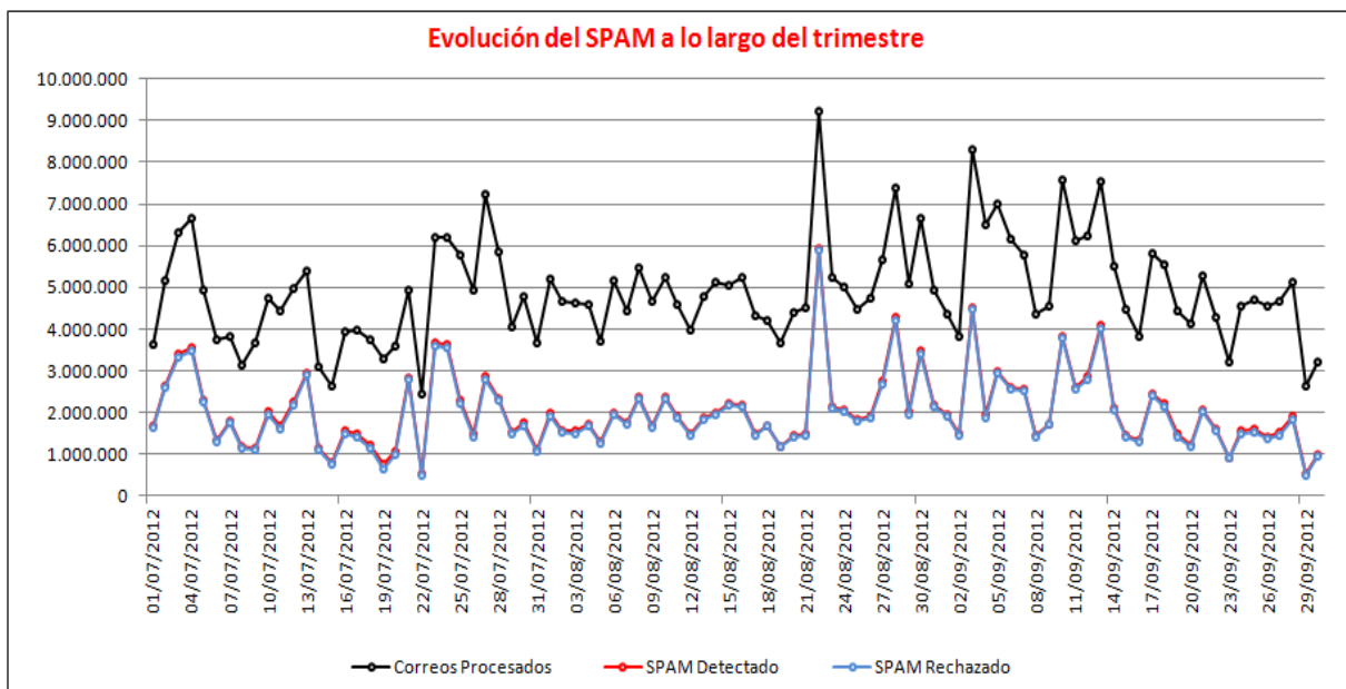
Figura 135: Evolución temporal del SPAM detectado por la red de sensores.
