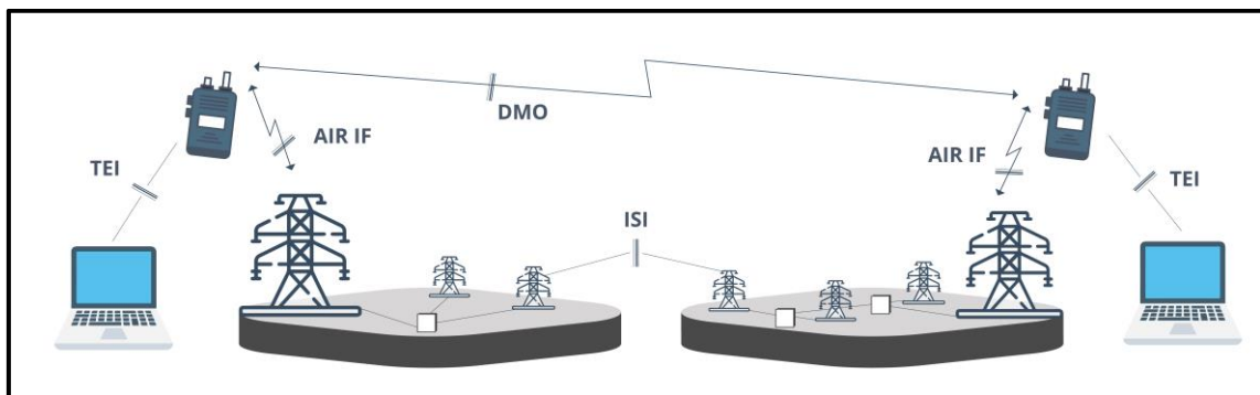
Ilustración 2: Arquitectura TETRA 3
